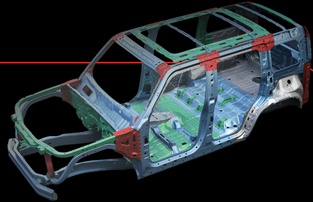
الأول من نوعه في فئة سيارات الطرق الوعرة قضيب مانع الانقلاب مدمج
