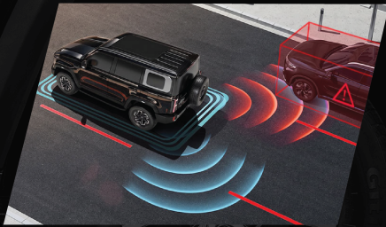
نظام المساعدة على تغيير المسار (LCA)
